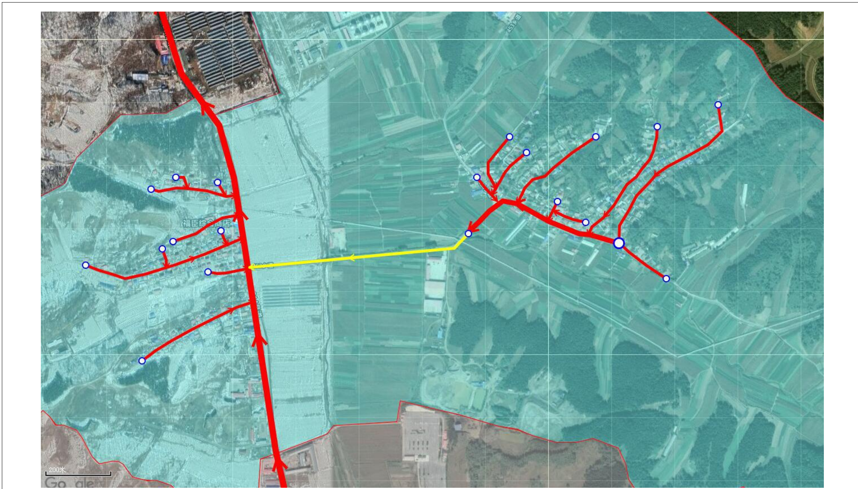
附图 8 丁家村污水管网规划
