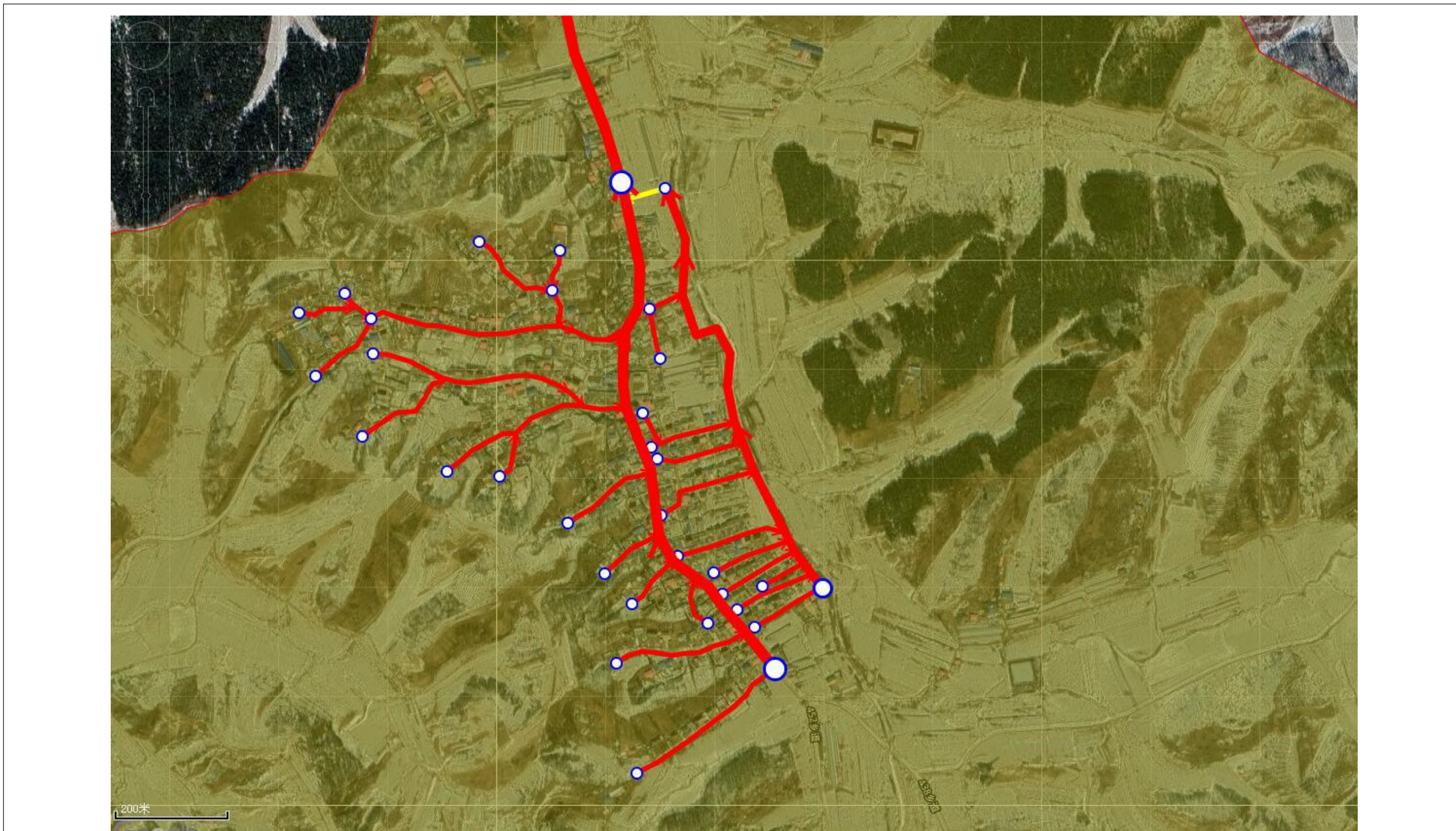
附图 10 英德村污水管网规划
