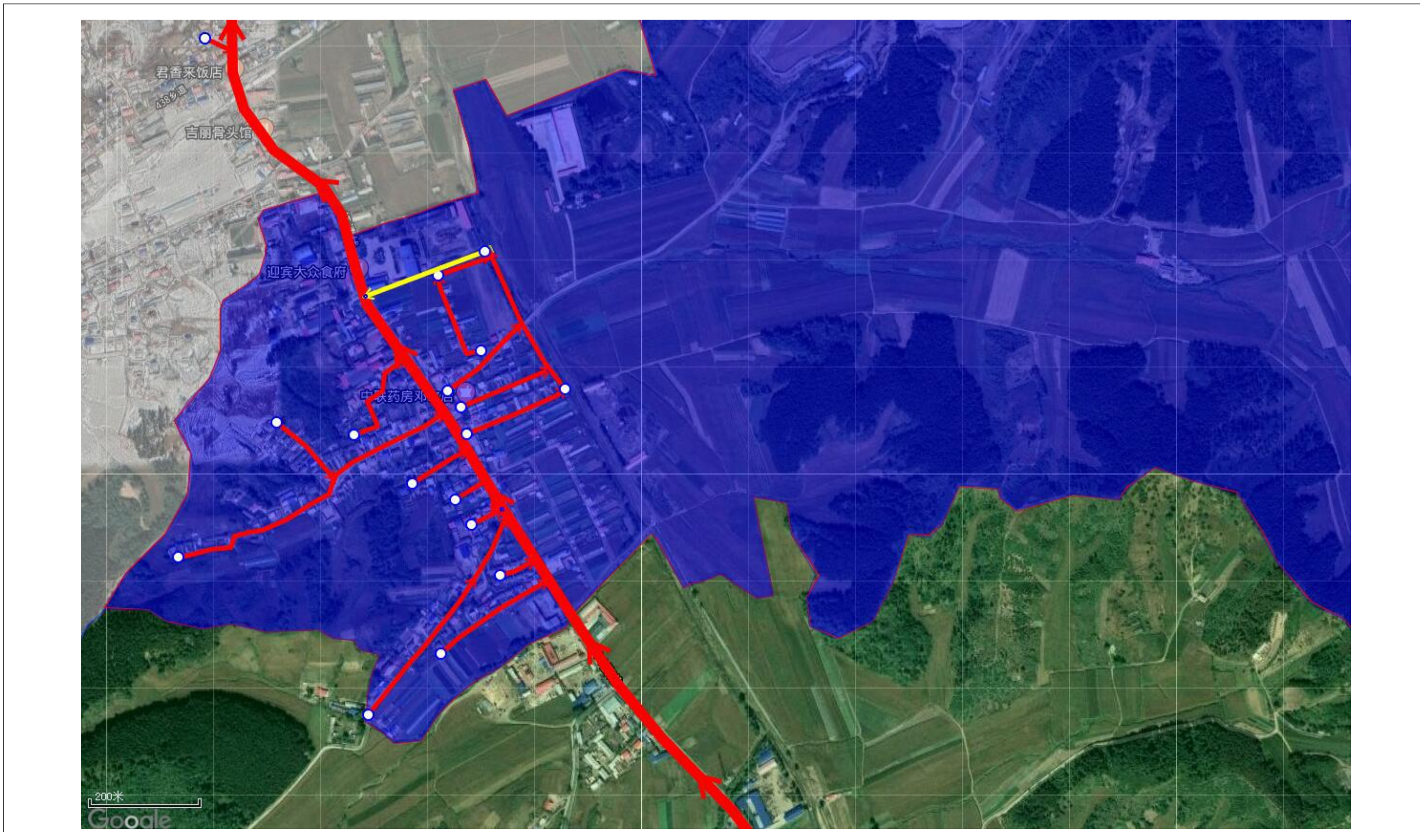
附图 5 前邓 1 村污水管网规划
