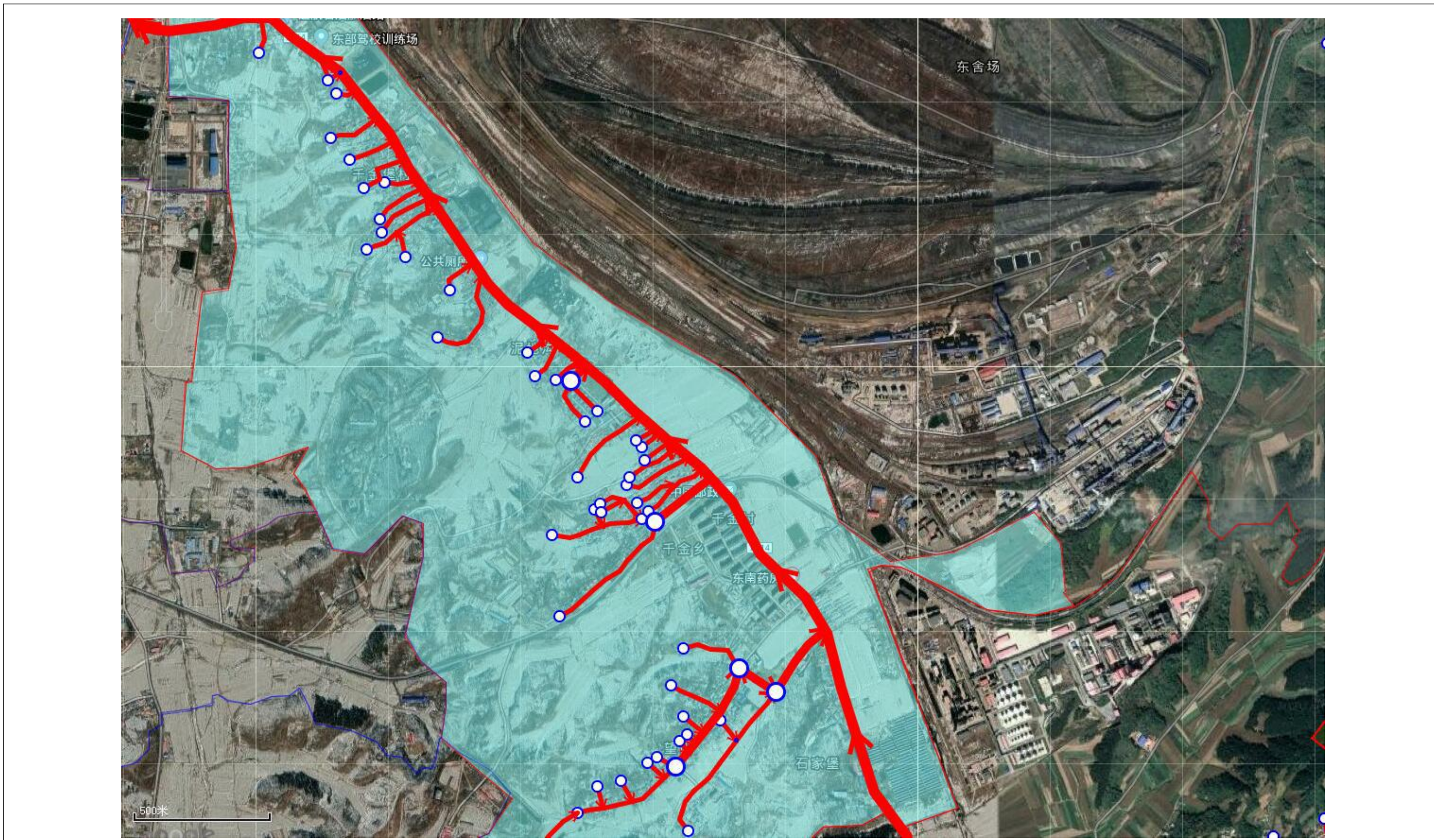
附图9 千金村污水管网规划
