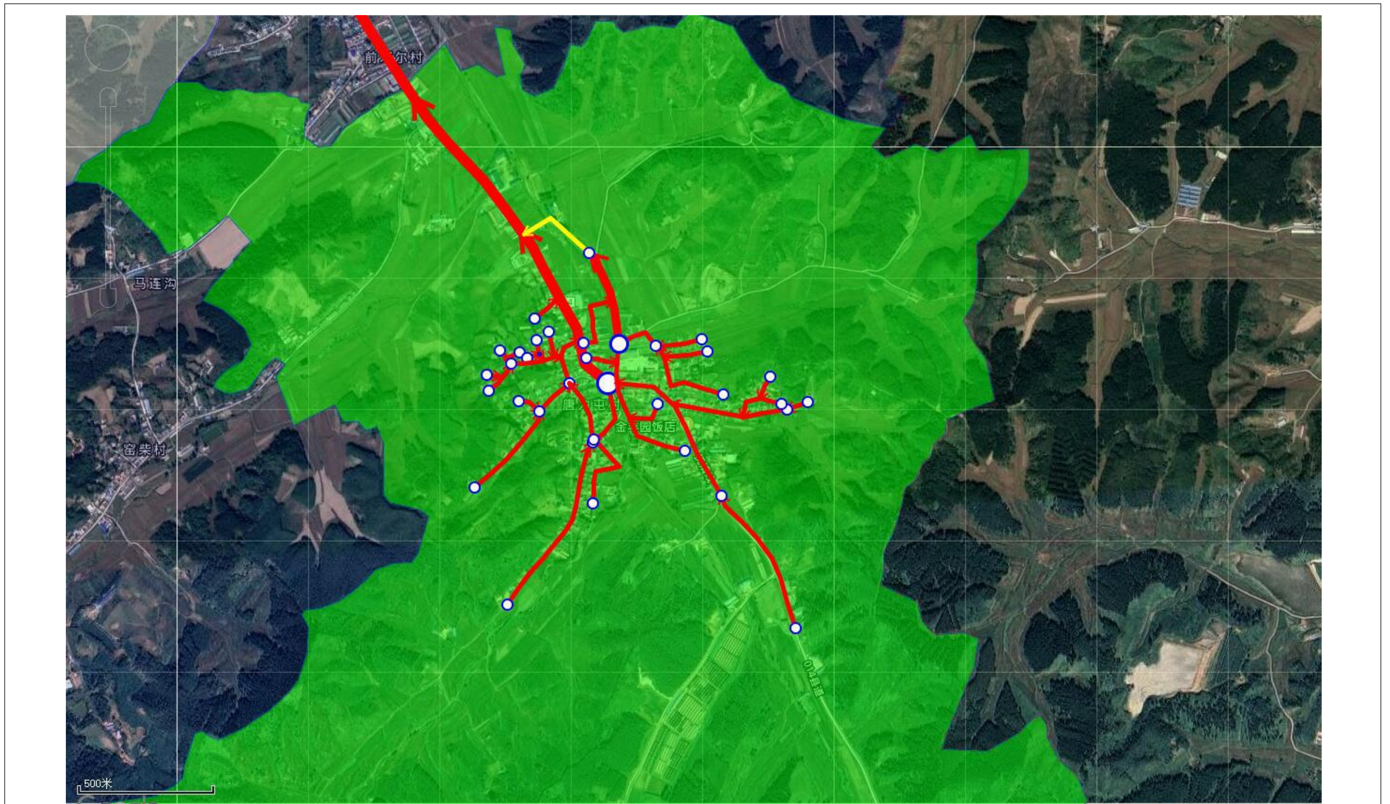
附图 4 唐力村污水管网规划
