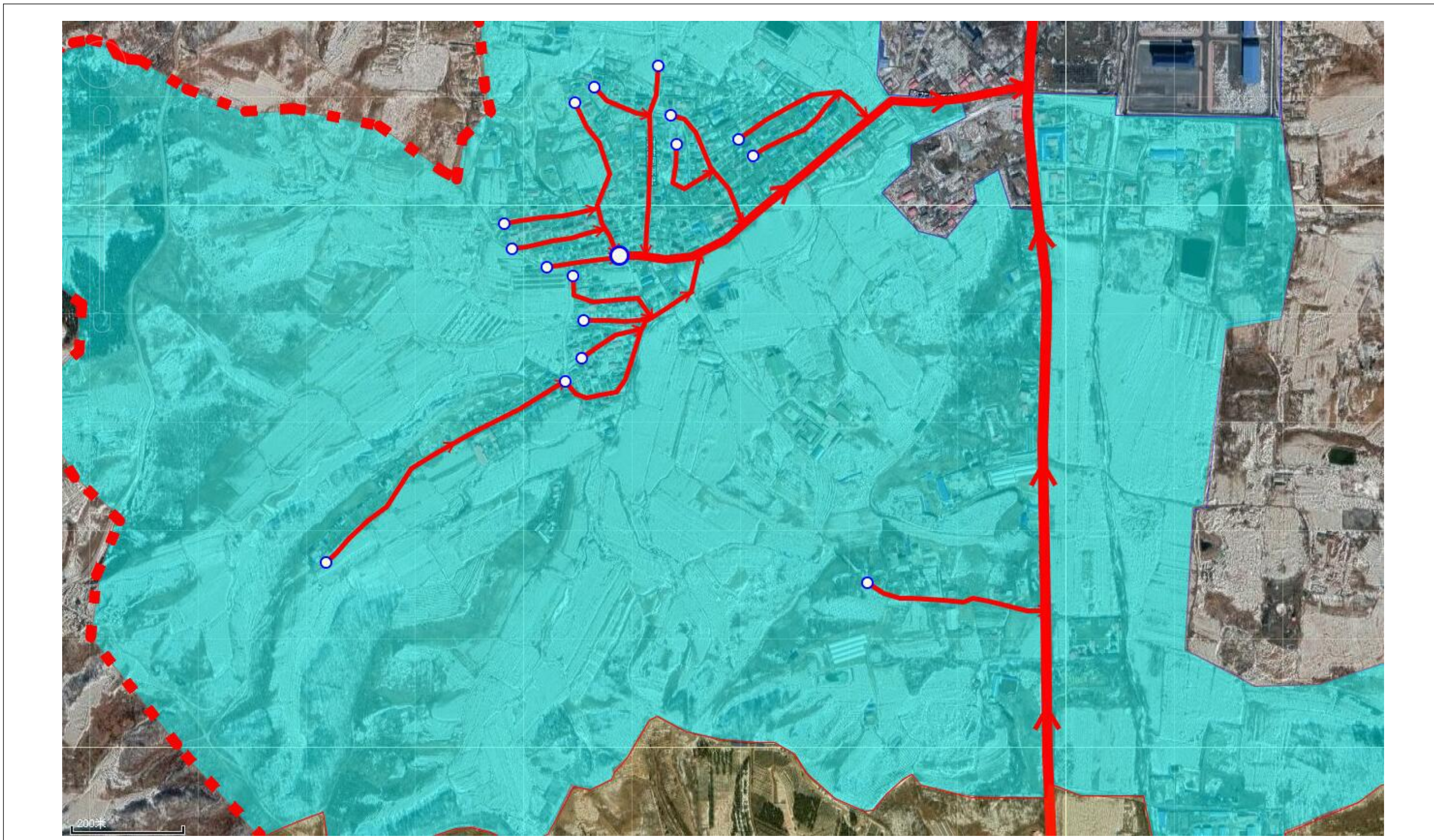
附图 12 荒地村污水管网规划
