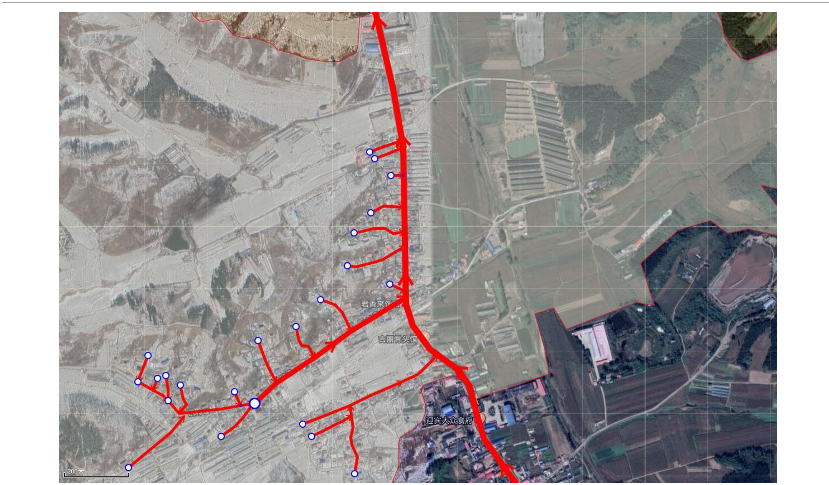
附图 7 后邓村污水管网规划
