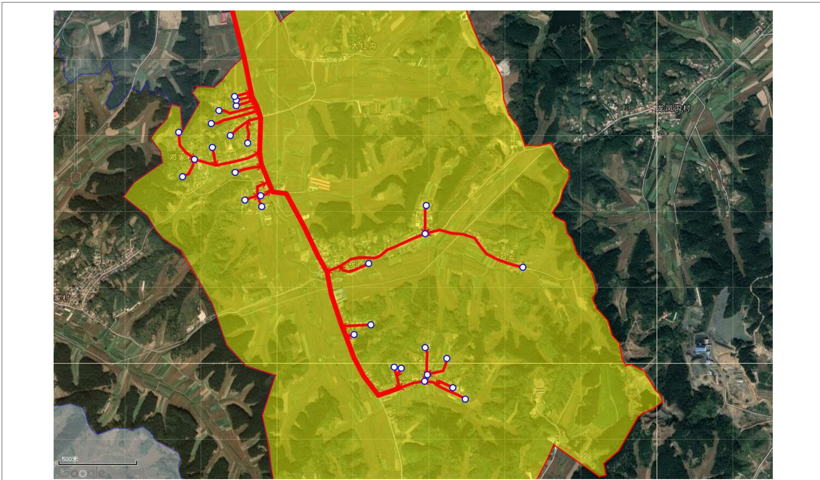
附图 2 高家村污水管网规划
